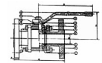
5. Valvola a sfera Bar stock turno regolare porto SS304 avvitato wp fino a 35 bar
