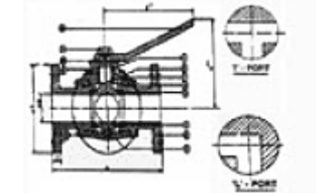
6. Valvola a sfera 3Way Corpo Pieno Alesaggio L o T porta fino a 100 wp bar
