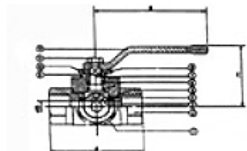
4. Valvola a sfera 3 pz rotonda regolare Porto Flangiate wp fino a 70 bar
