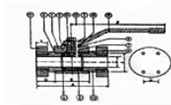
2. Valvola a sfera Round corpo regolare porto Flangiate wp fino a 70 bar
