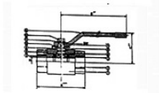
1. Válvula de bola Forjado quadrado corpo único pc Full Bore lixada até 550 bar
