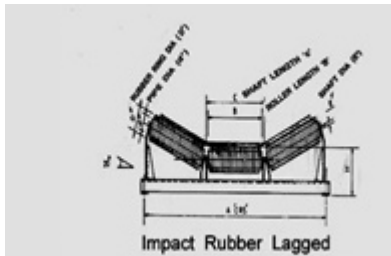
Impacto desfasado rolos de borracha
